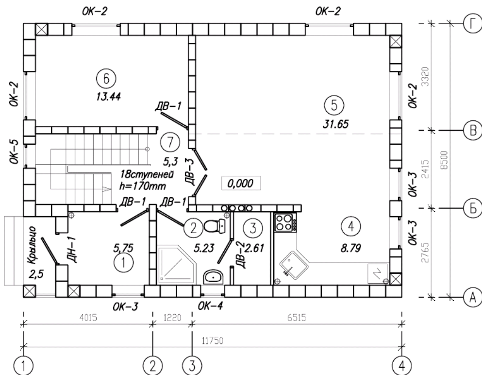
Экспликация 1-го этажа
