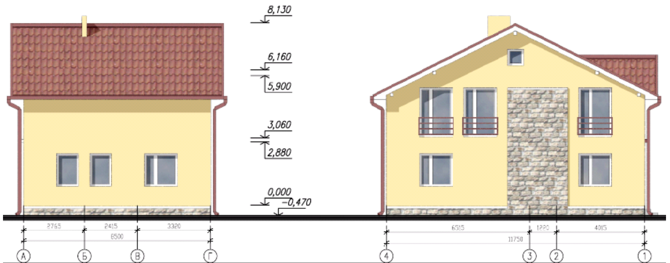
Фасад в осях А-Г М 1:100
