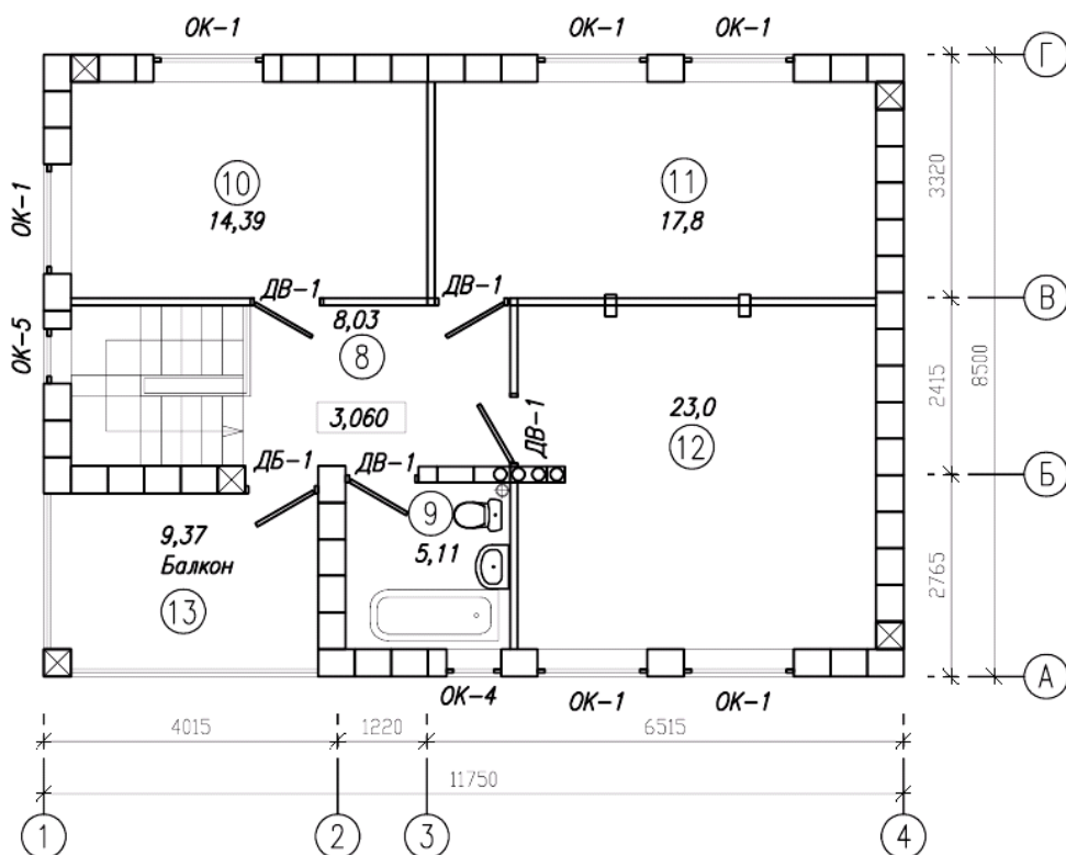
Экспликация 2-го этажа
