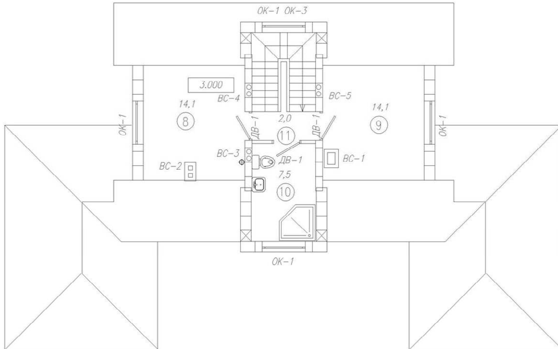
Экспликация 1-го этажа
