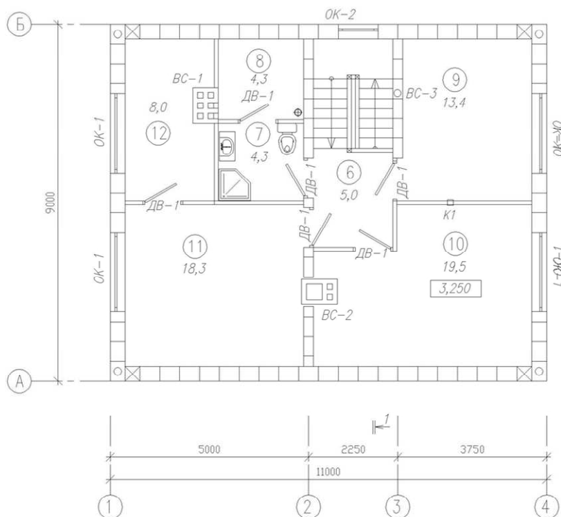
Экспликация 1-го этажа
