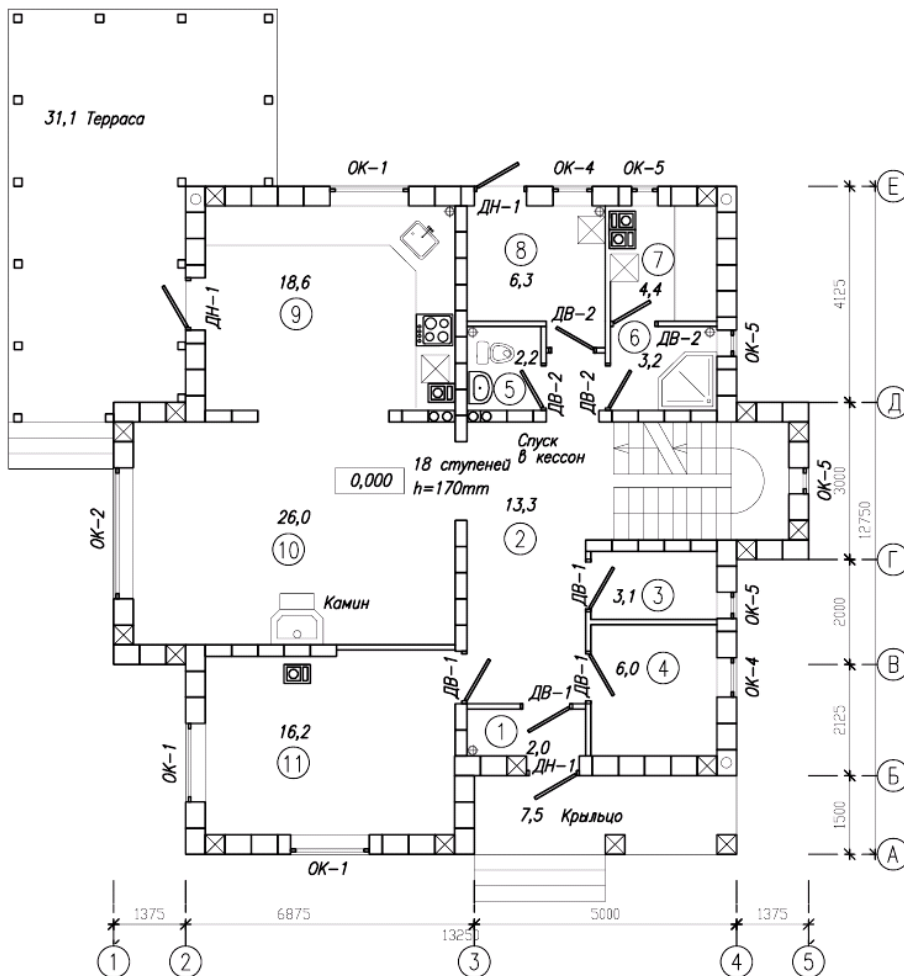
Экспликация 1-го этажа
