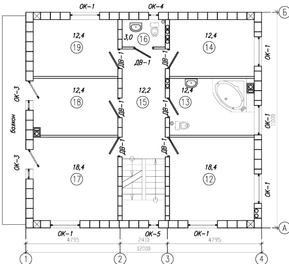
Экспликация 2-го этажа
