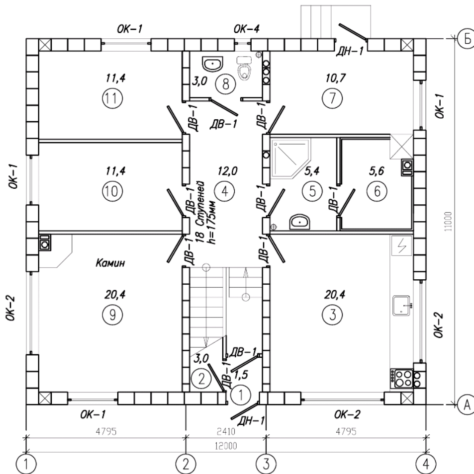
Экспликация 1-го этажа
