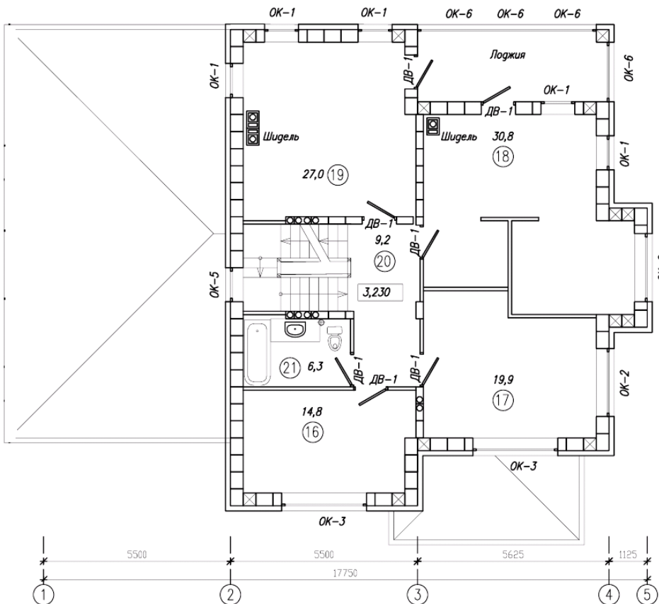
План 2-го этажа
