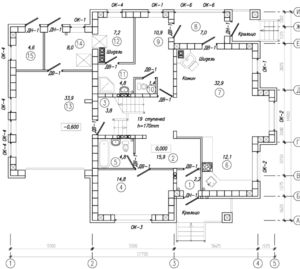
Экспликация 1-го этажа
